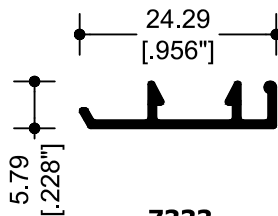
7333 MOSQUITERO
