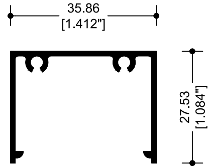
29076 BOLSA LISA
