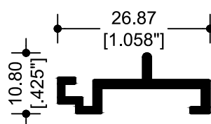
9966 ADAPTADOR MOSQUITERO
