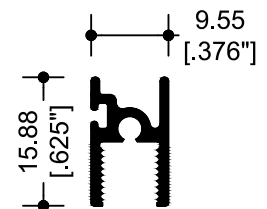
10575 ZOCLO
