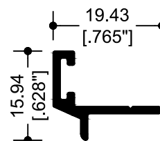
10220 ADAPTADOR OXXO
