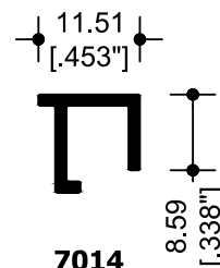
7014 JUNQUILLO
