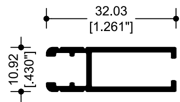
53358 ZAPATA
