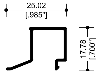
74635 JUNQUILLO ESTRECHO
