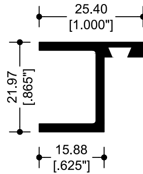
7102 BATIENTE
