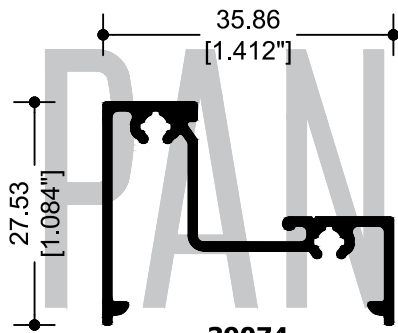
39074 ESCALONADO
