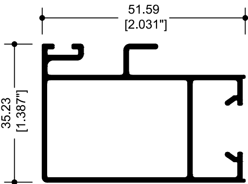
67848 TRASLAPE PUERTA
