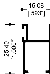
11836 CERCO
