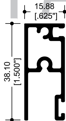
10358 MOSQUITERO
