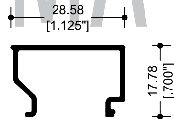
73978 JUNQUILLO ANCHO
