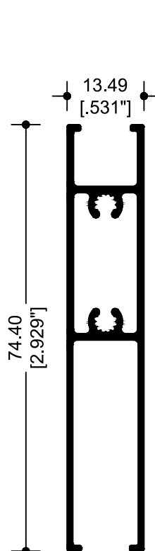
37825 ZOCLO PUERTA
