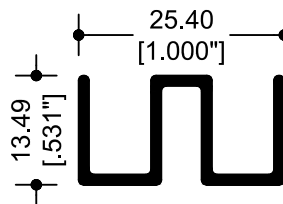
63329 GUÍA
