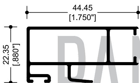
69955 TRASLAPE PUERTA
