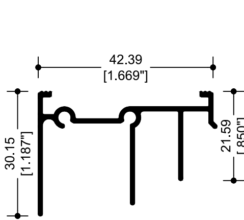
10568 CABEZAL
