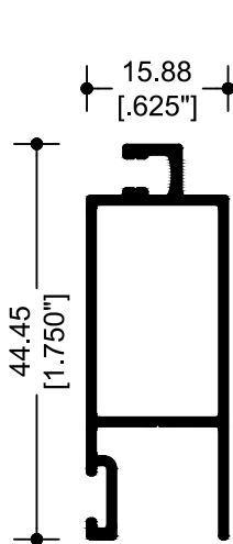
66534 CERCO MOSQUITERO
