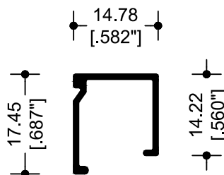
36370 JUNQUILLO
