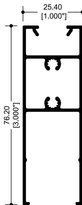
67842 ZOCLO
