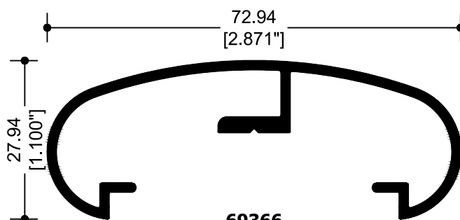
69366 PASAMANOS 3"
