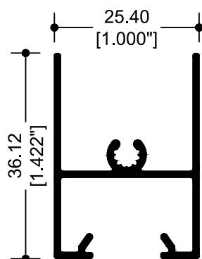
67836 CABEZAL
