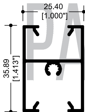
69082 INTERMEDIO
