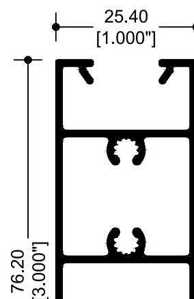
67835 ZOCLO VENTANA
