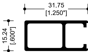
8320 CERCO VENTANA
