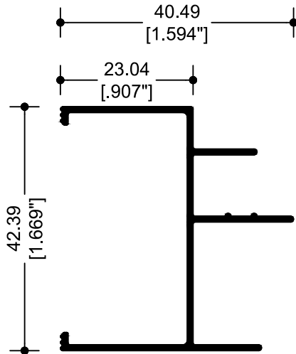
10570 JAMBA
