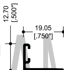
11032 BATIENTE
