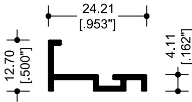
67013 BASE
