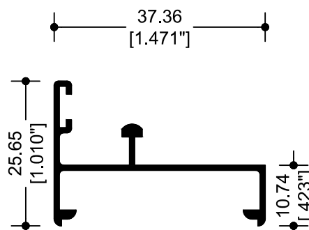
11838 RIEL
