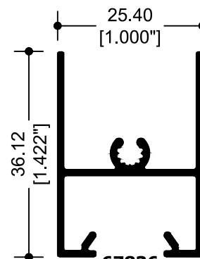
67836 CABEZAL VENTANA
