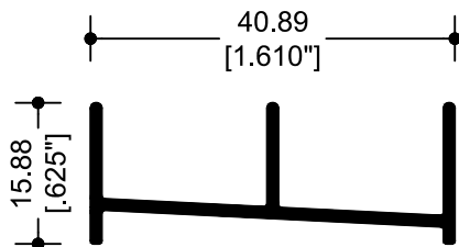
10198 RIEL INFERIOR
