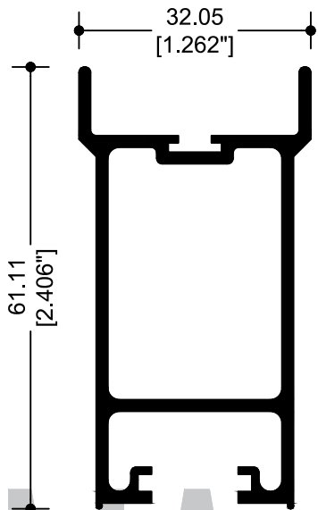
67850 CERCO OXXO
