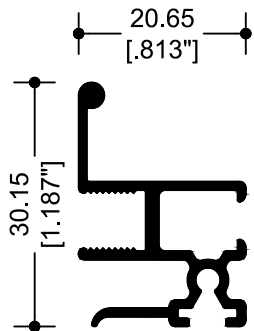
10571 CERCO MÓVIL
