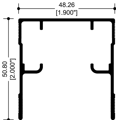
9947 RIEL SUPERIOR
