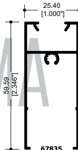
67835 ZOCLO VENTANA
