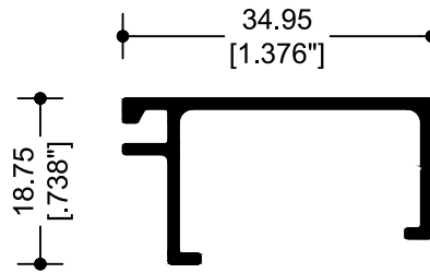
28939 JUNQUILLO
