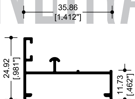
15310 RIEL
