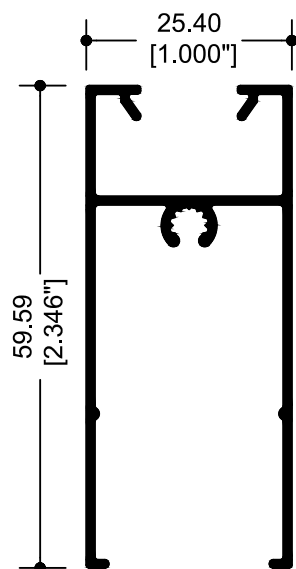
67835 ZOCLO
